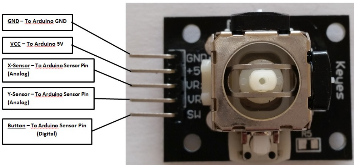
Abbildung 2: Pin-Belegung
