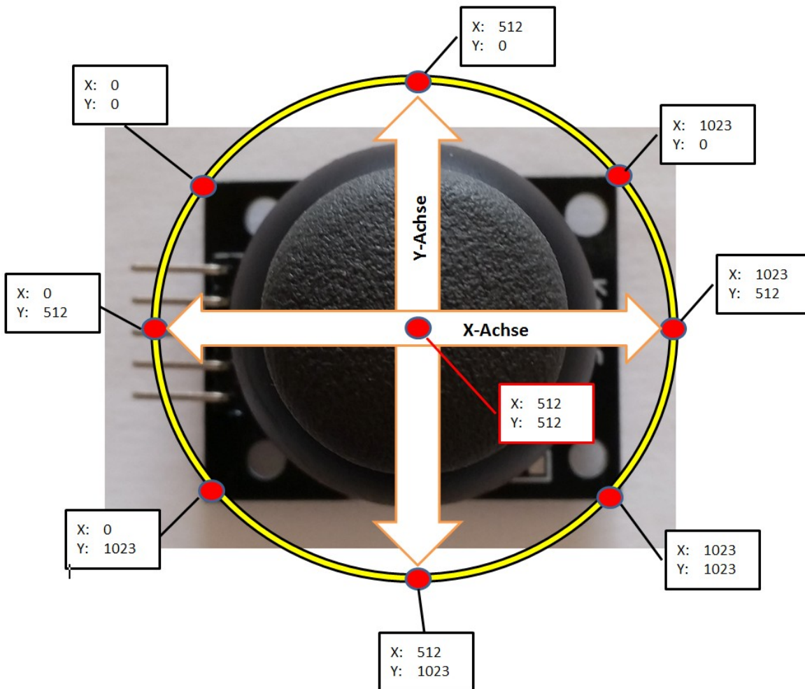
Abbildung 1: Joystick-Koordinaten
